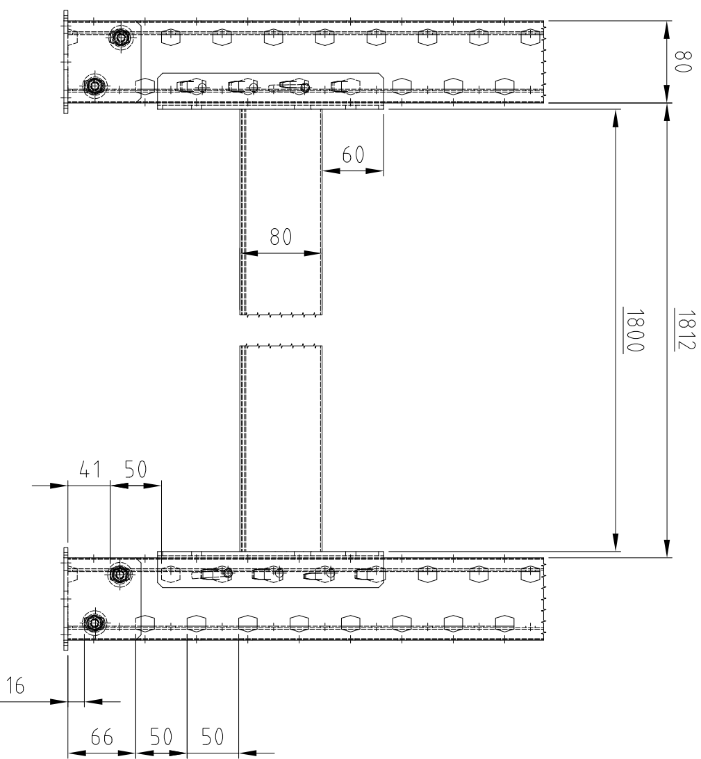
Draufsicht
